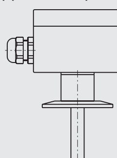
Clamp pipe connection per DIN 32676
